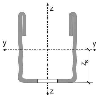
Bild 4: Kennwerte des U-Profiles 53 mit Lochung \varnothing 8 mm nach Anlage A, Seiten 3 und 6
