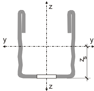
Bild 6: Kennwerte des U-Profils 60 mit Lochung \square 20 \times 40 \text{ mm} nach Anlage A, Seiten 6, 71 und 141
