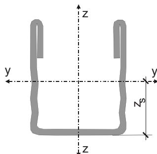
Bild 2: Kennwerte des U-Profiles 53 ohne Lochung nach Anlage A, Seiten 3 und 6
