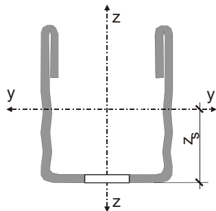
Bild 3: Kennwerte des U-Profiles mit Lochung \varnothing 12 mm nach Anlage A, Seiten 3 und 6
