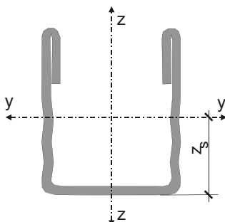
Bild 5: Kennwerte des U-Profiles 60 ohne Lochung nach Anlage A, Seiten 6, 71 und 141
