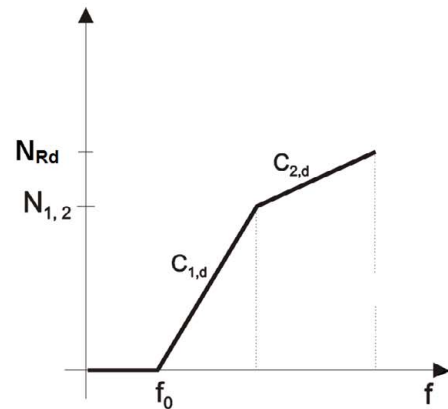
Bild 9: trilineare Federkennlinie
