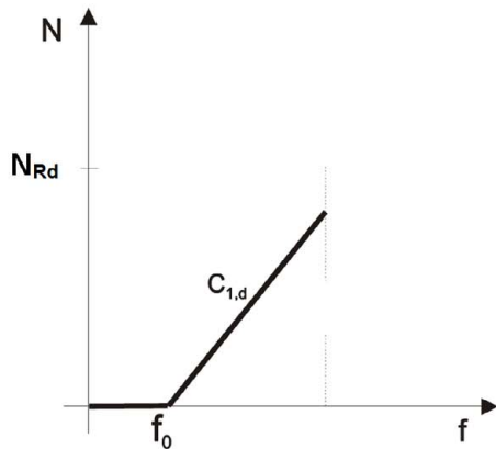
Bild 8: bilineare Federkennlinie
