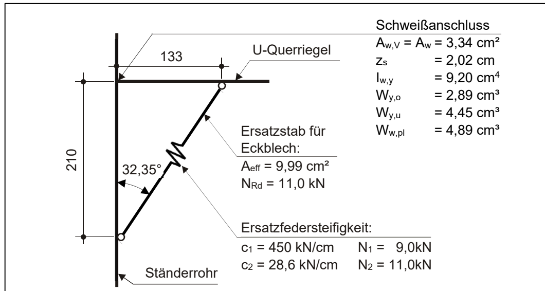
Bild 1: Kennwerte des Eckblechs
